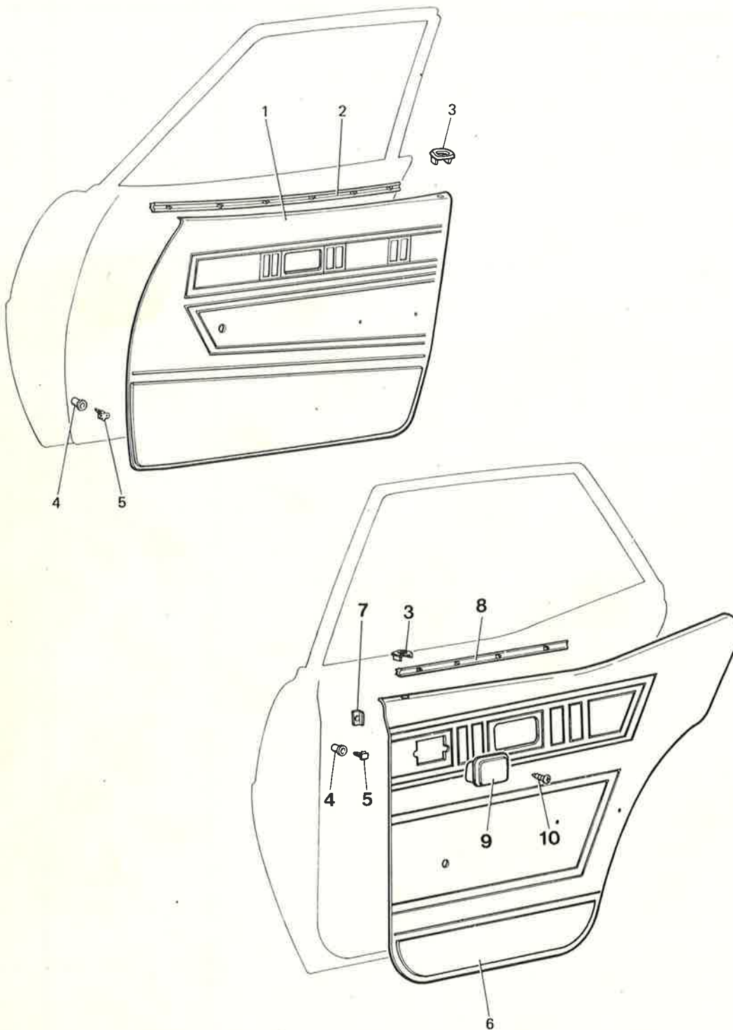
DOOR TRIM
